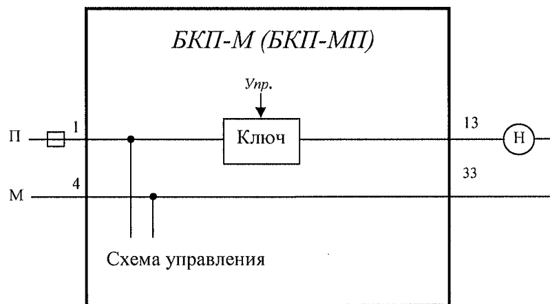
Рисунок 1.5 – Схема подключения контрольного реле
