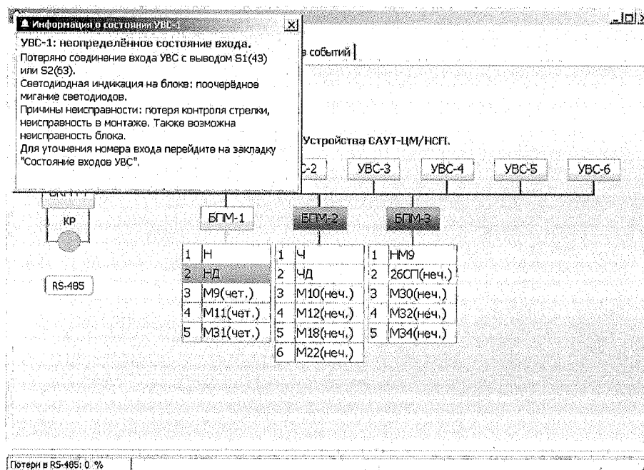
Рисунок 2.6 – После щелчка кнопкой мыши на элементе УВС-1
