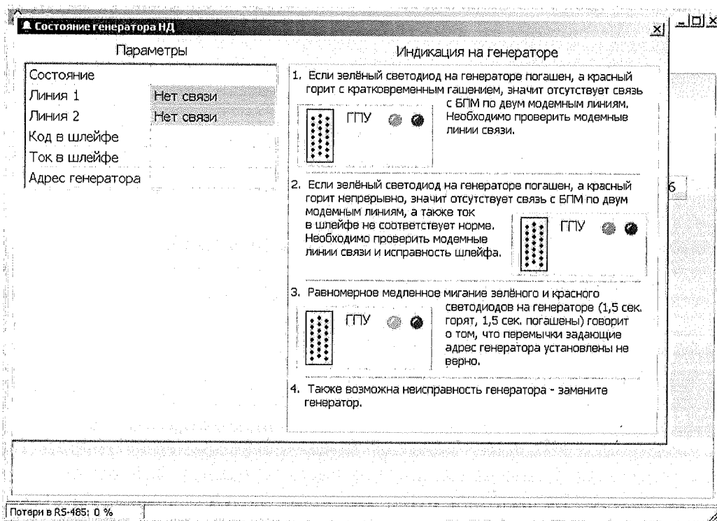
Рисунок 2.8 – После щелчка кнопкой мыши на генераторе «НД»
