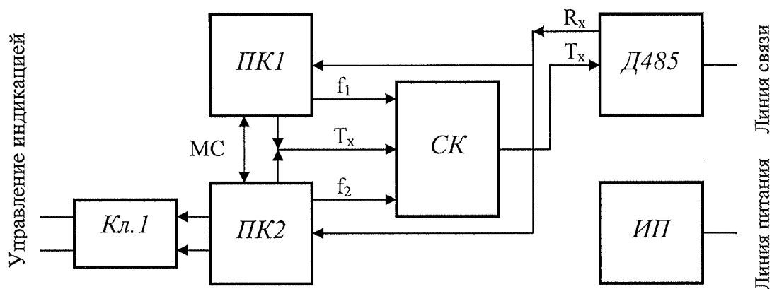
Рисунок 1.4 – Структурная схема БКП-М
